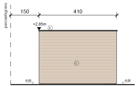
ZICHT ACHTERGEVEL
