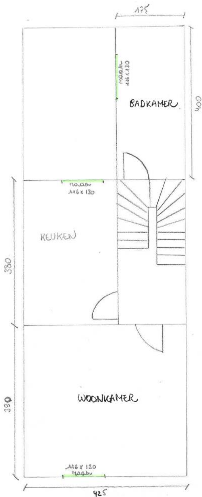
GRONDPLAN - EERSTE VERDIEPING SCHAAL : 1/50 Bestaande toestand
