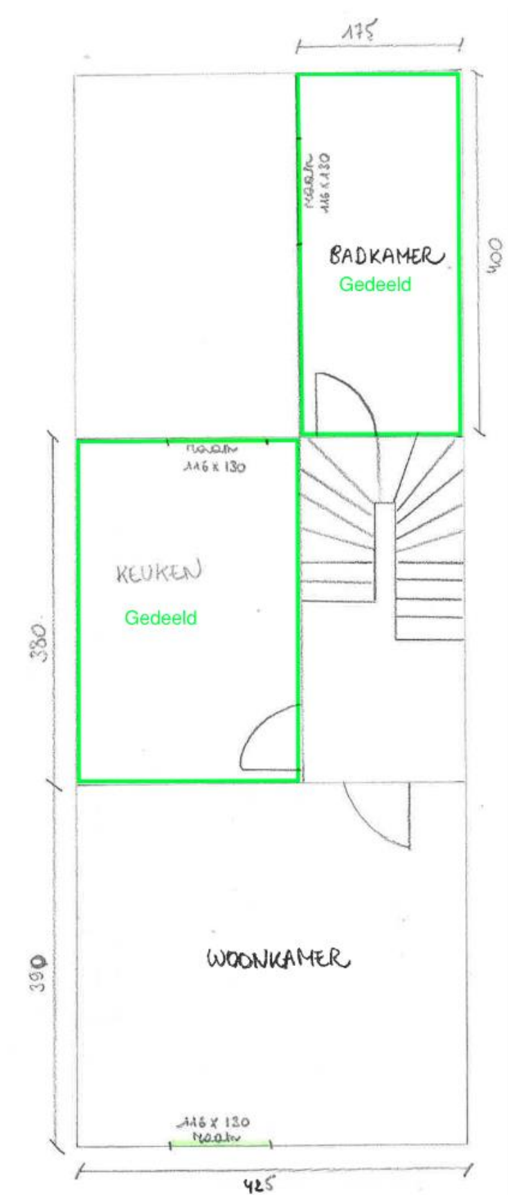
GRONDPLAN - EERSTE VERDIEPING SCHAAL : 1/50 Nieuwe toestand
